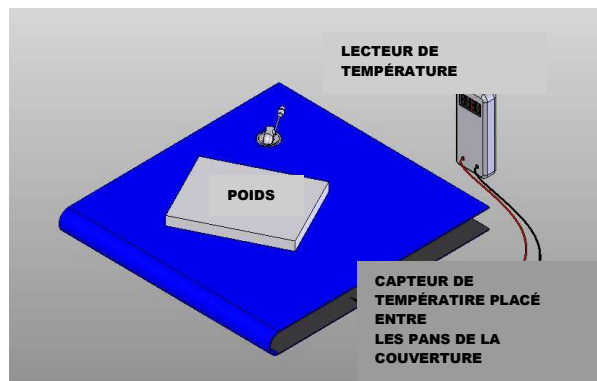
Illustration 3 : Configuration de test de la couverture chauffante
